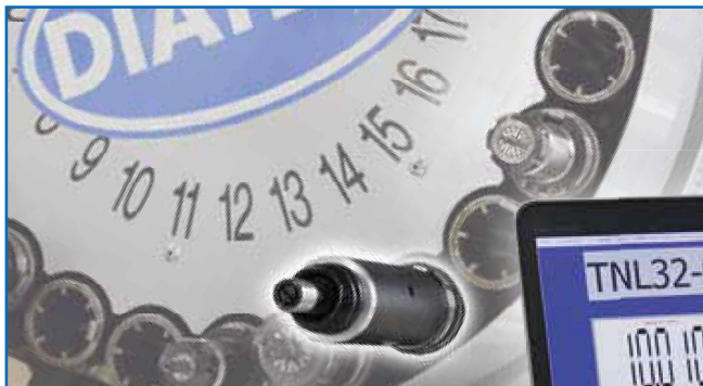
BMD im Werkzeug-Wechselsystem Plug gauge BMD in tool changing system
